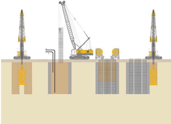
Diaphragm wall ( wharf)
